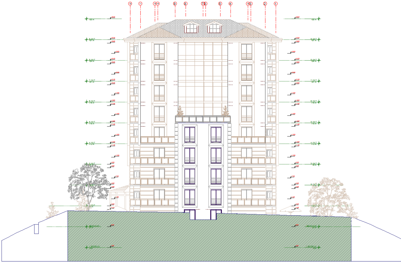
ARKA CEPHE Ö: 1/50
